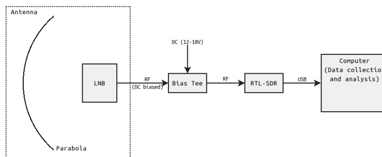
Fig: Acquisition chain [28].
